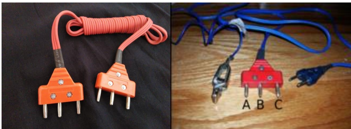
Foto derecha: pasante de florete / sable; de izquierda a derecha pinza cocodrilo, conexión a rulo, conexión a arma. Foto izquierda: pasante de espada.
